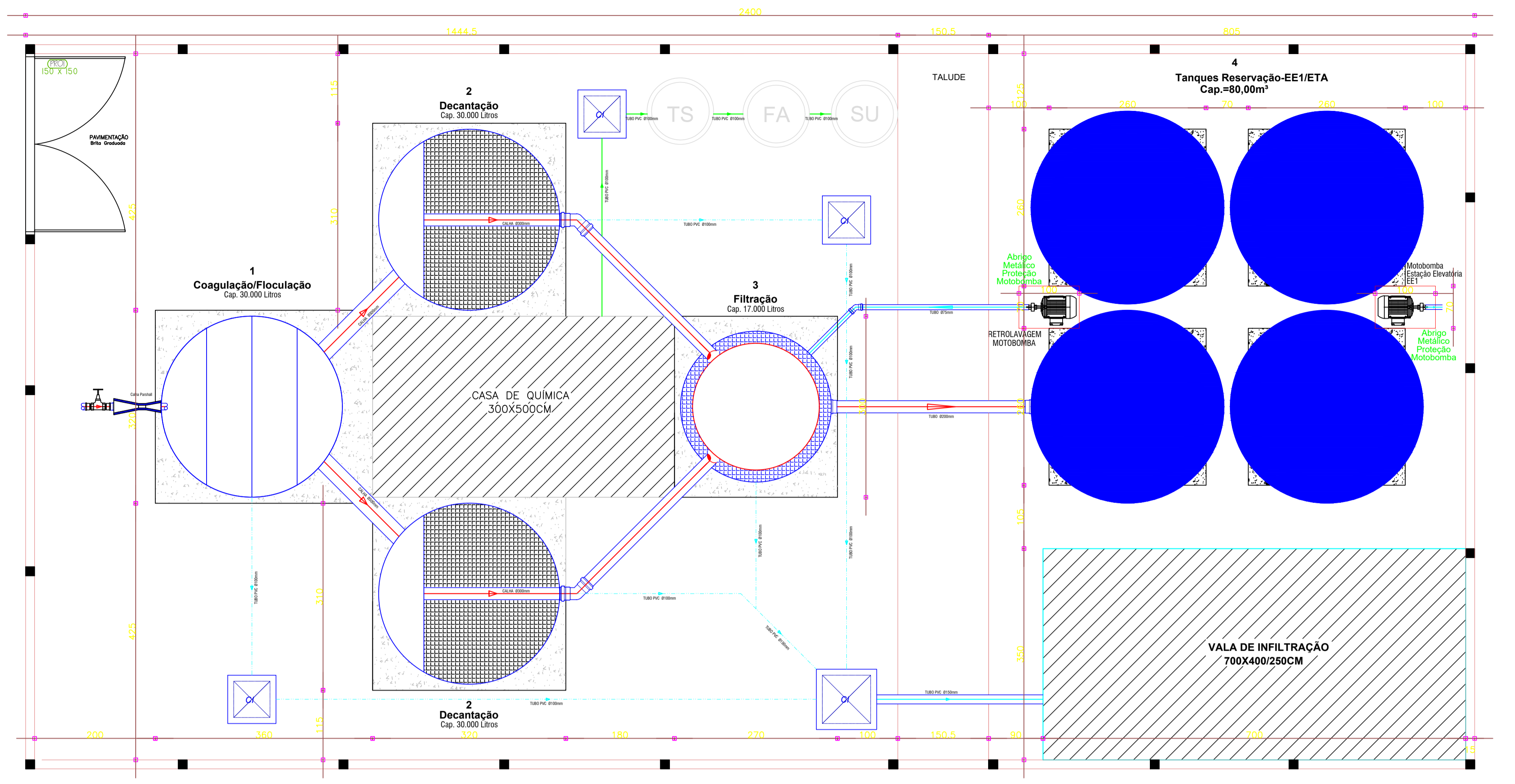
PLANTA BAIXA ETA A = 288,00m 2 E = 1/50
