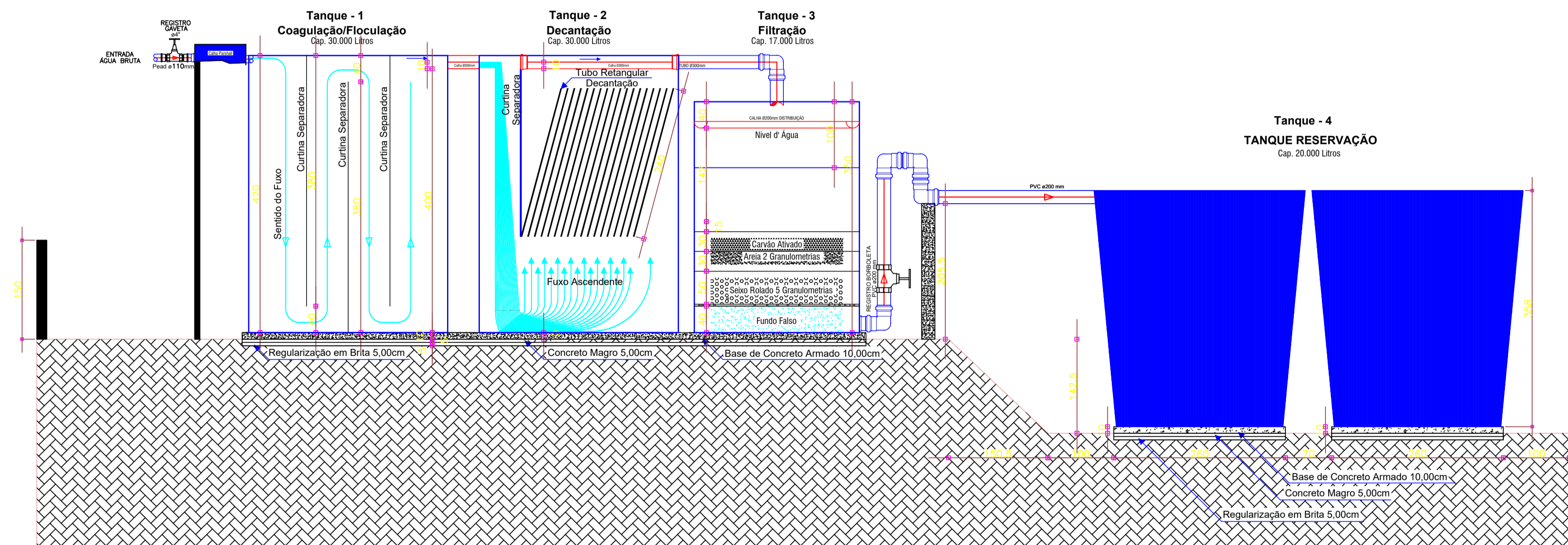
ELEVÇÃO ESTAÇÃO DE TRATAMENTO - ETA E = 1/50
